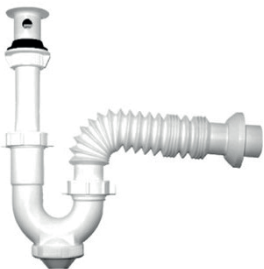
Trampa completa para Lavabo Rugo
